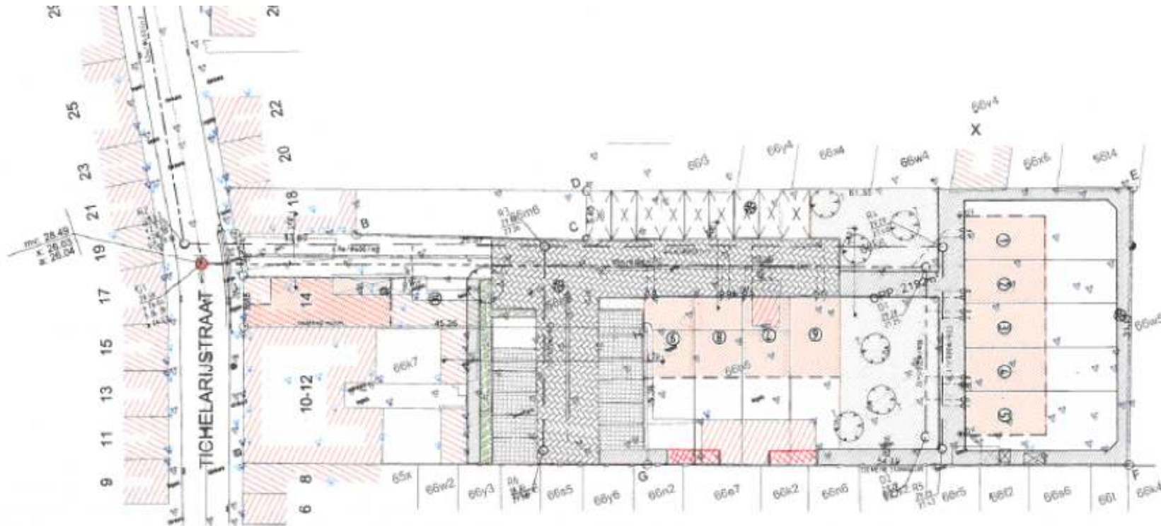
TURNHOUT - INBREIDING TICHELARIJSTRAAT Grondplan ontworpen toestand infrastructuur Schaal 1:100
