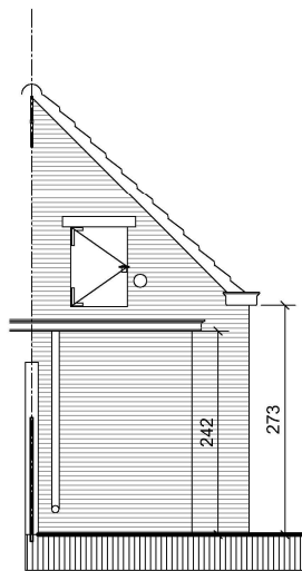
ACHTERGEVEL AANBOUW
